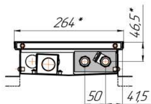
Разрез
