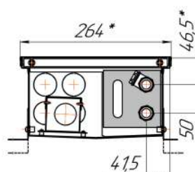
Разрез
