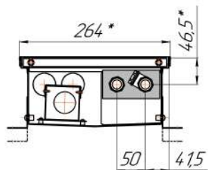
Разрез
